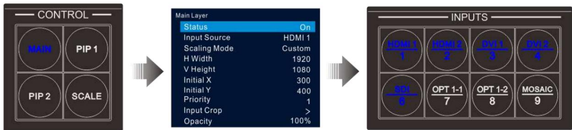
Figura 5-12 Sorgenti di input del livello di commutazione
