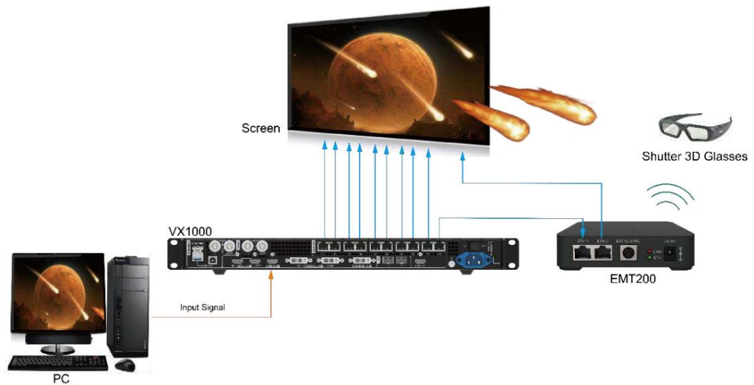
Figura 5-38 Connessioni 3D
