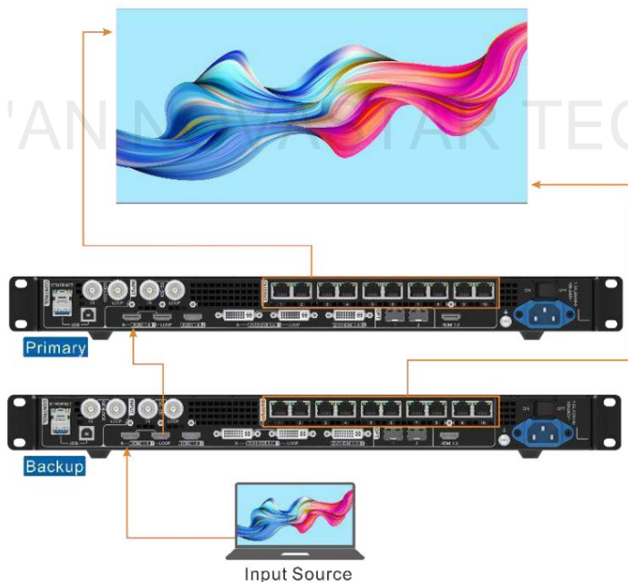
Figura 5-25 Connessione di backup del dispositivo
