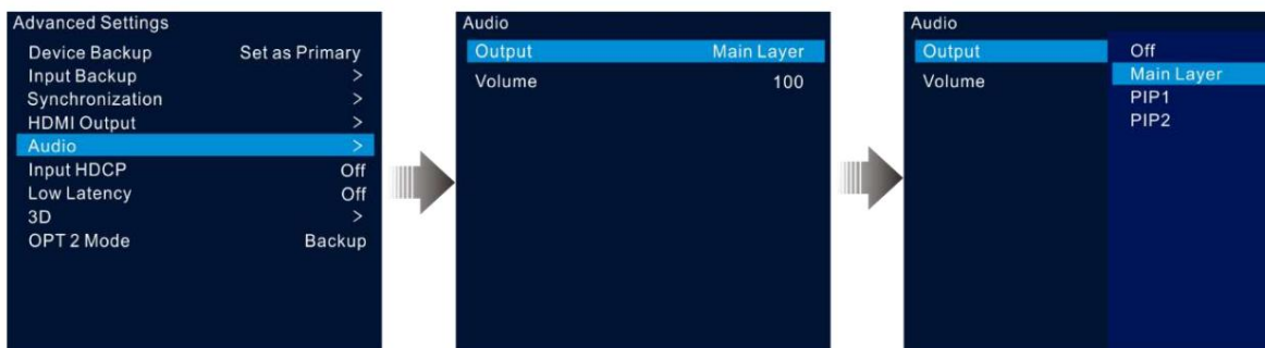
Figura 5-37 Uscita audio
