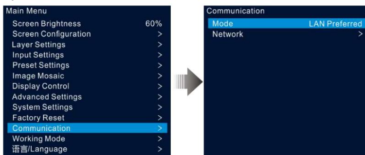
Figura 5-47 Modalità di comunicazione
