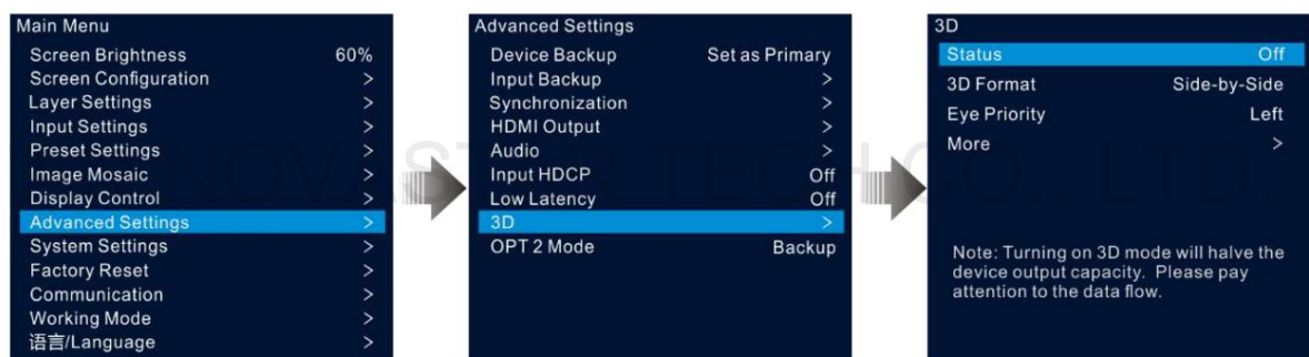
Figura 5-39 Impostazioni 3D
